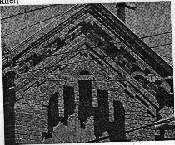
Щипец
